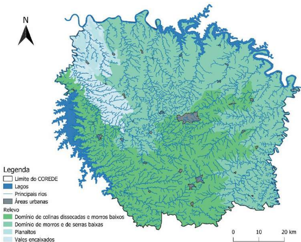
Figura 22 - Regiões fisiográficas do Corede Norte
