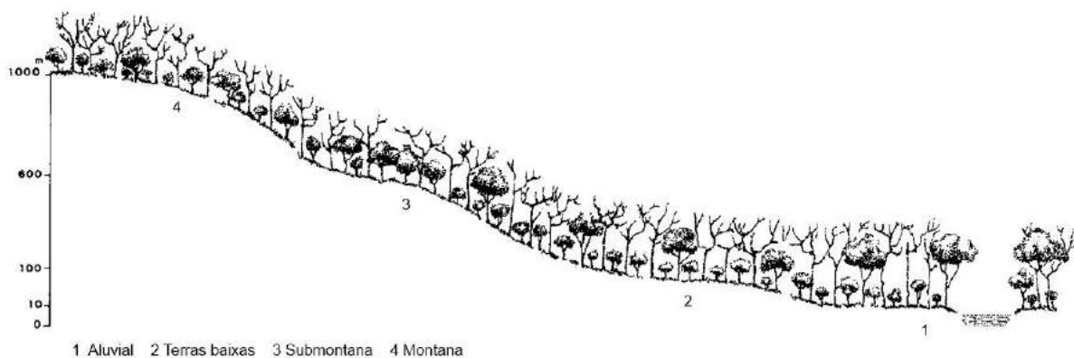
Figura 33 - Perfil esquemático da Floresta Estacional Decidual – FED
