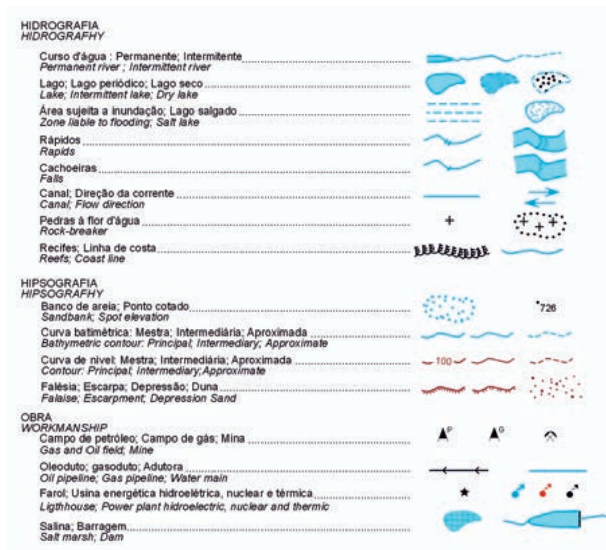
Figura 3: Principais convenções cartográficas utilizadas na representação do espaço geográfico
