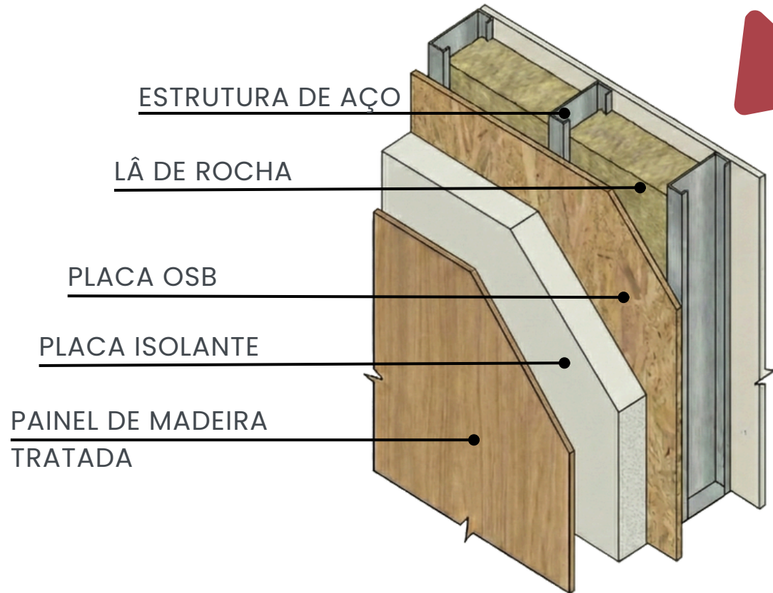
FIGURA 43: FECHAMENTOS E REVESTIMENTOS: STEELFRAME
