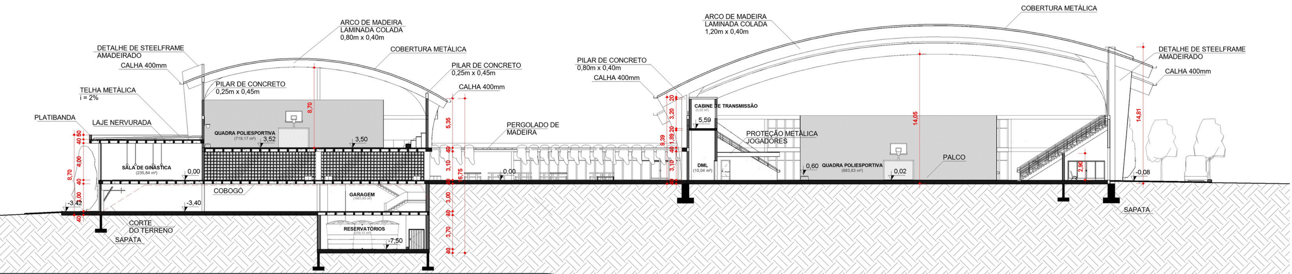
CORTE B'B'' 1/200
