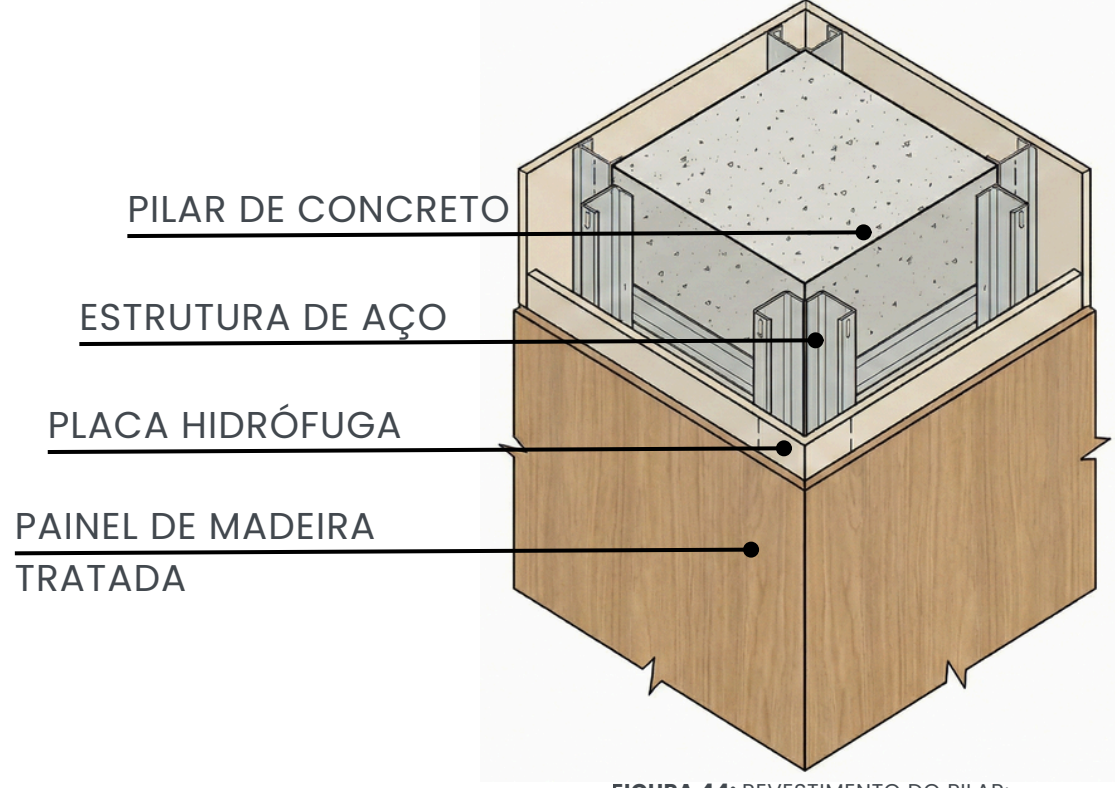
FIGURA 44: REVESTIMENTO DO PILAR: STEELFRAME
