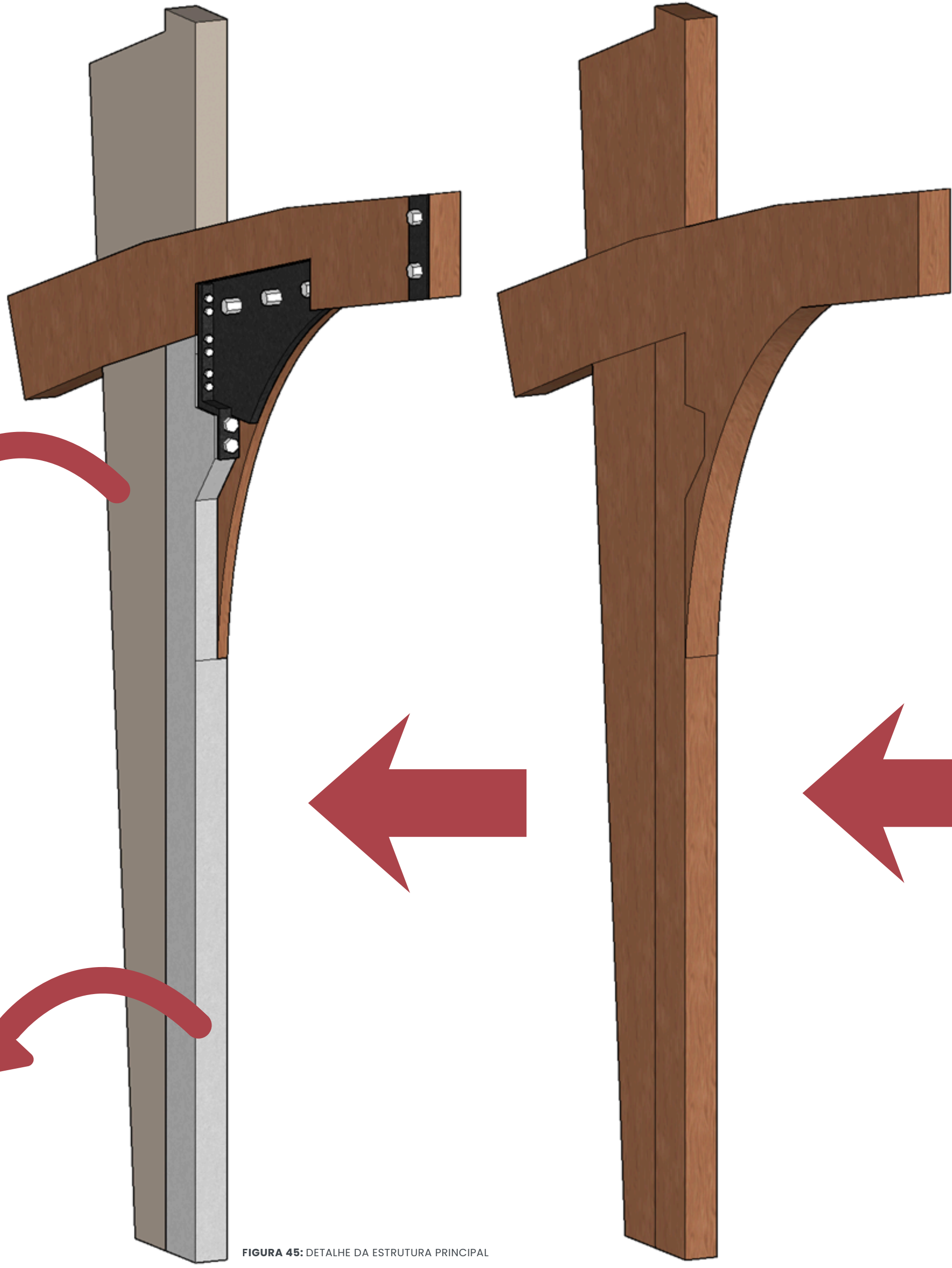
FIGURA 45: DETALHE DA ESTRUTURA PRINCIPAL
