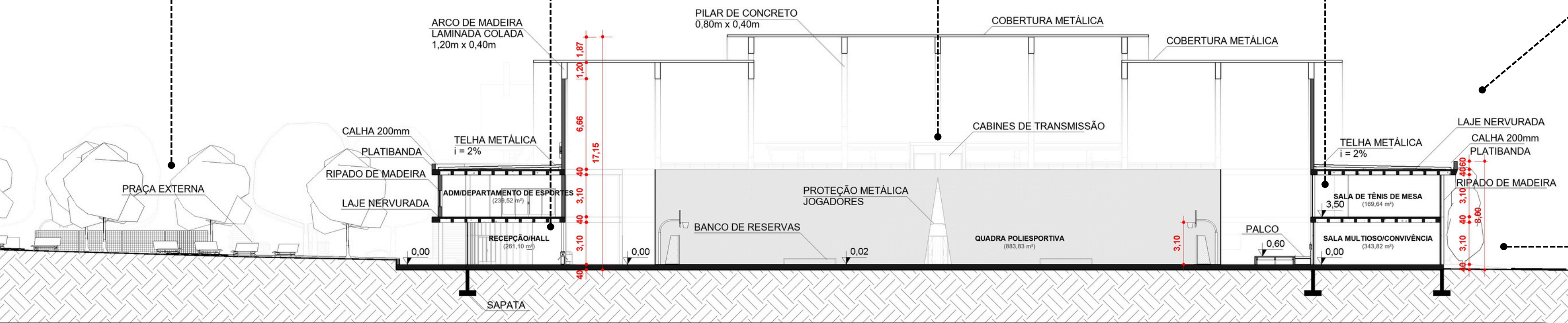
CORTE C'C'' 1/200
